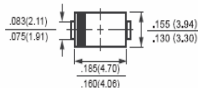
SMB (DO-214AA)
